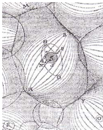
Рис. 3.3.12. Вихри тонкой материи по представлению Декарта. В центре находится Солнечная система (Oeuvres de Descartes, v. IX)
